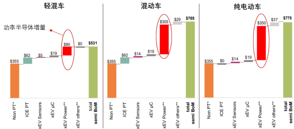
图 21：2019 不同等级电动汽车平均半导体含量（红色部分为功率半导体）
