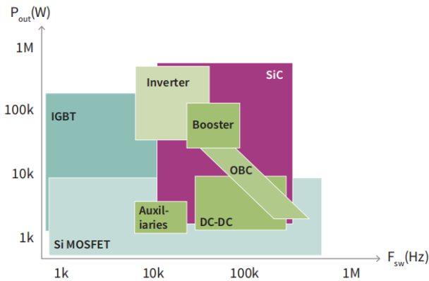
图 57：SiC 功率器件能满足大部分电动车核心部件需求
